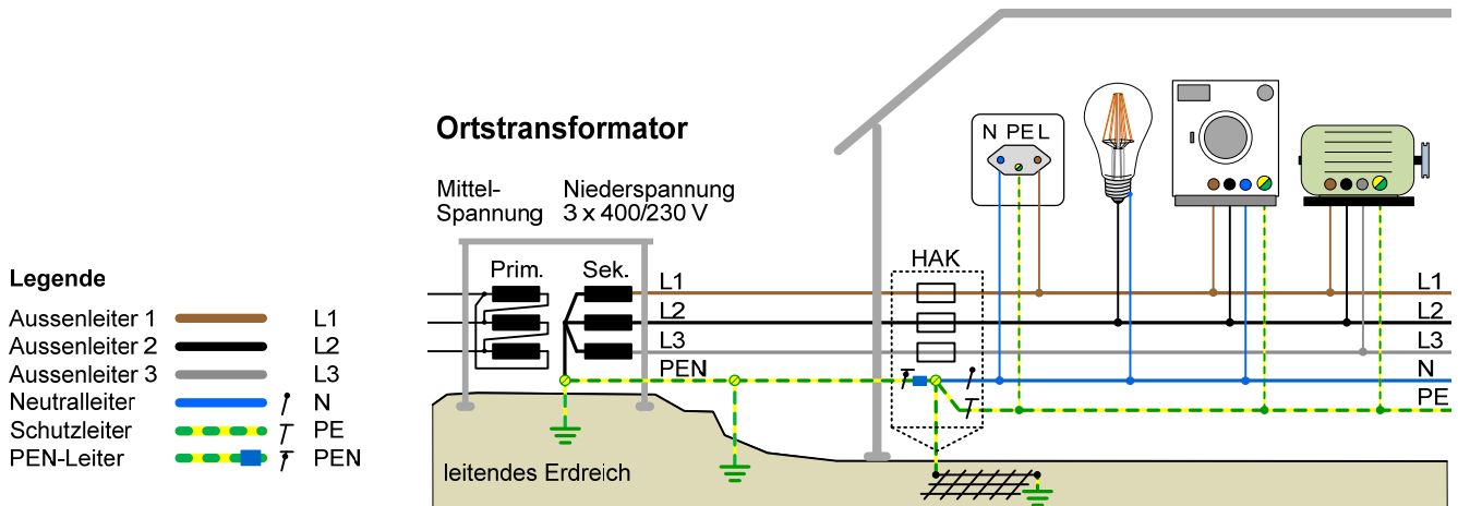
Ortstransformator
