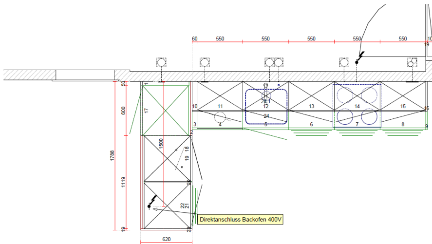
Grundriss
